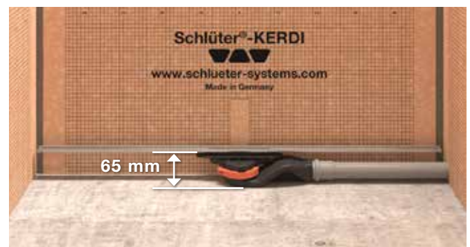
Altura constructiva reducida: 65 mm
